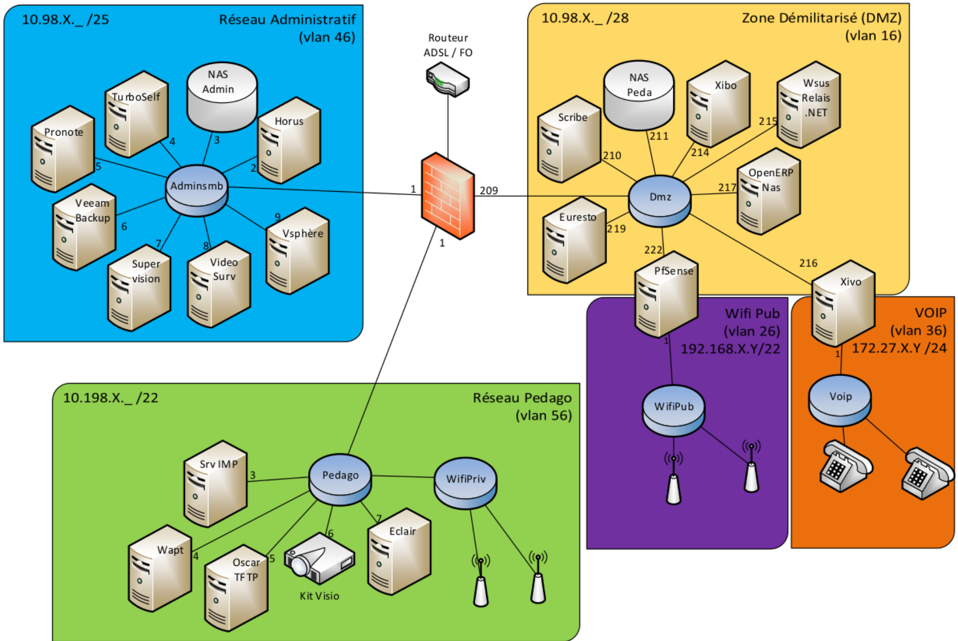
Structure de l'environnement réseau d'un établissement - Schéma niveau 1, les serveurs
